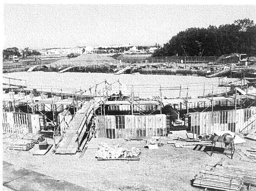
建設中の沼ノ端室内スケートリンク
