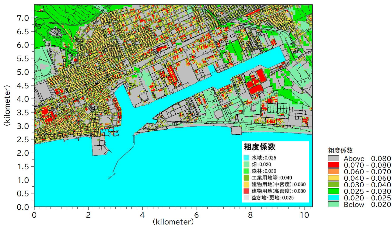
図- 9 10m 格子領域粗度データの例(苫小牧西港周辺)
