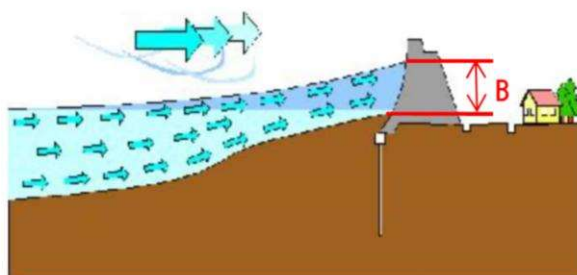
図2 吹き寄せ効果
