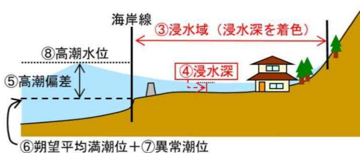
図3 高潮水位等の定義
