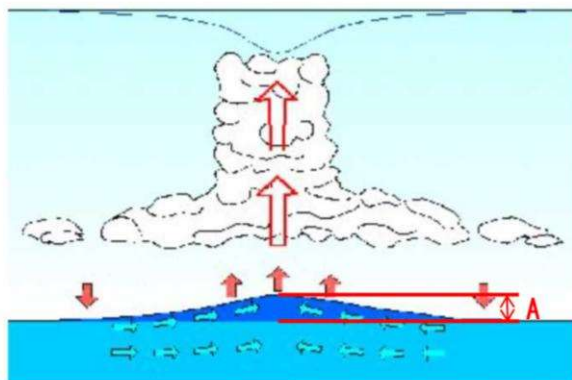
図1 吸い上げ効果
