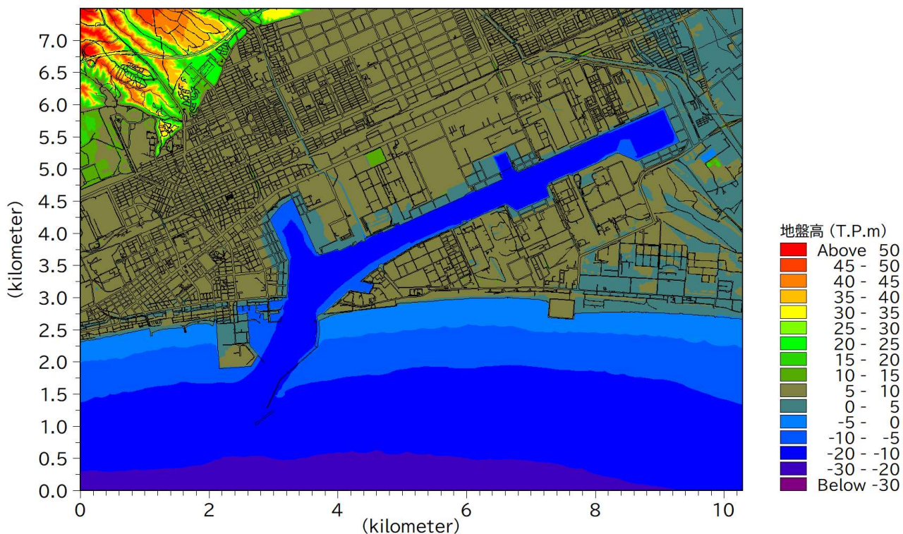
図- 8 10m 格子領域地形データの例(苫小牧西港周辺)
