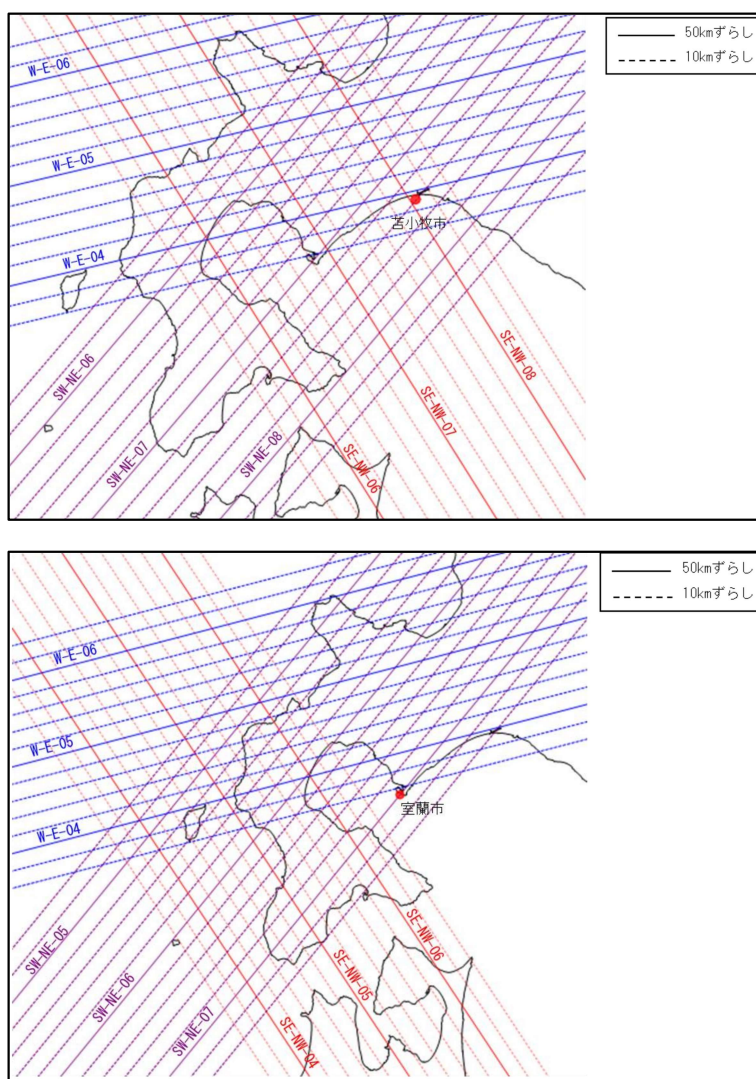
図-3 想定台風の検討経路(上:苦小牧東港、下:室蘭港)
