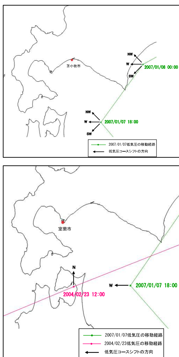
図- 4 想定する低気圧の検討経路(2007/01/07 低気圧および 2004/02/23 低気圧)
