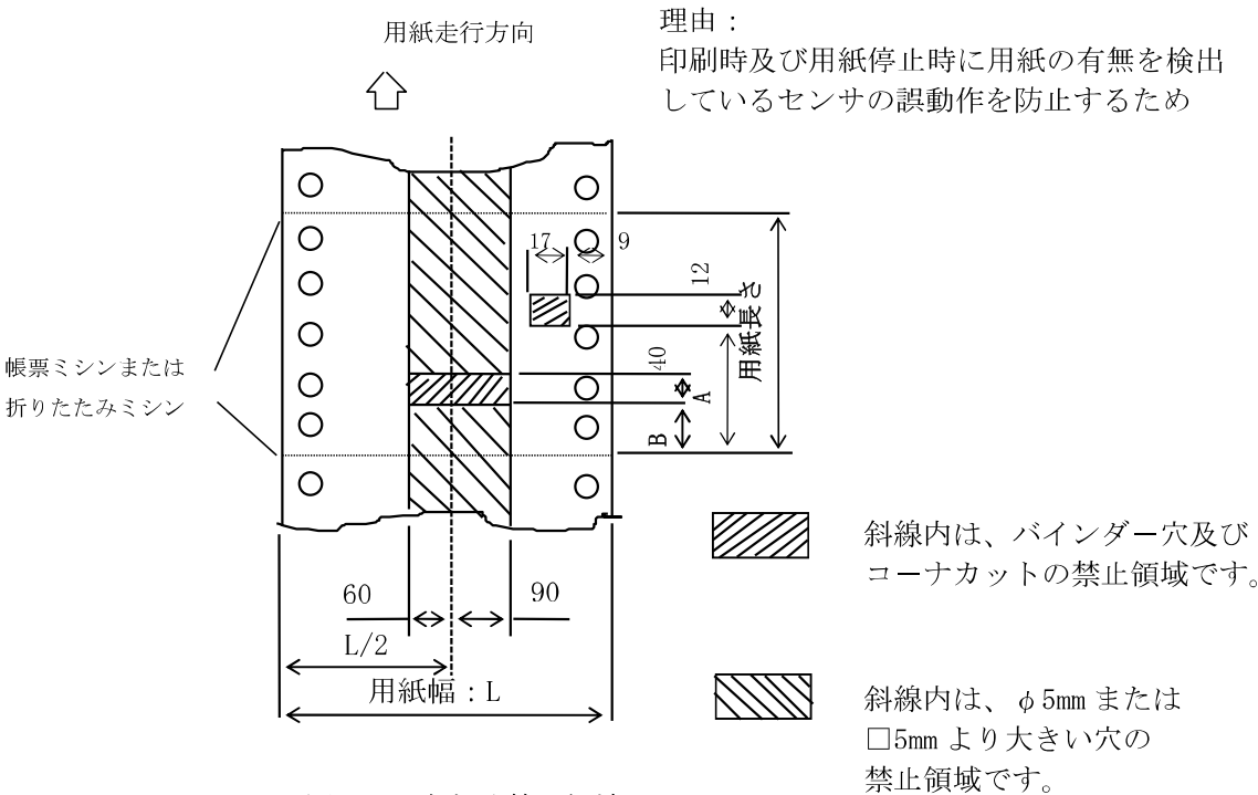
図 B-6 穴あけ禁止領域
