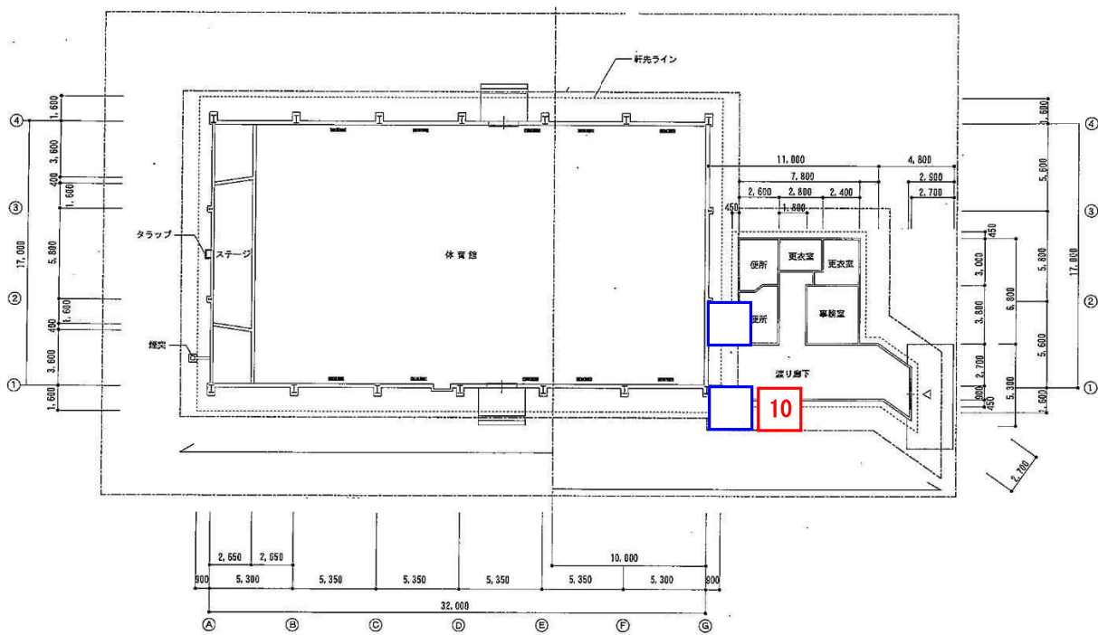
日吉体育館平面図
