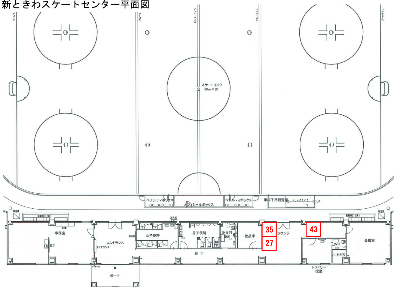
新ときわスケートセンター平面図
