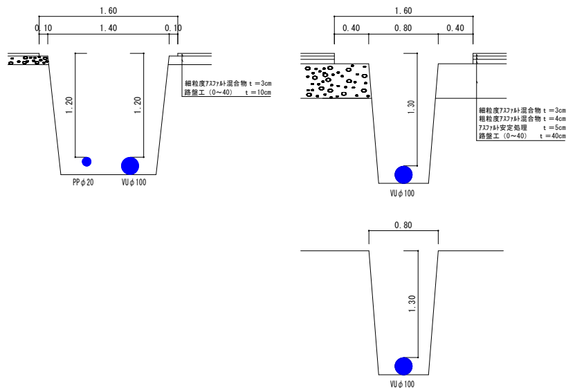
土工定規図 1:40
