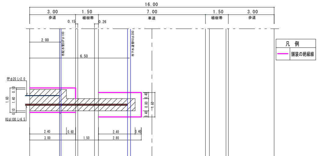
平面図 1:100
