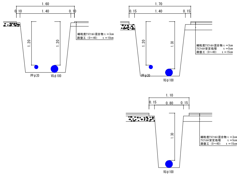
土工定規図 1:40
