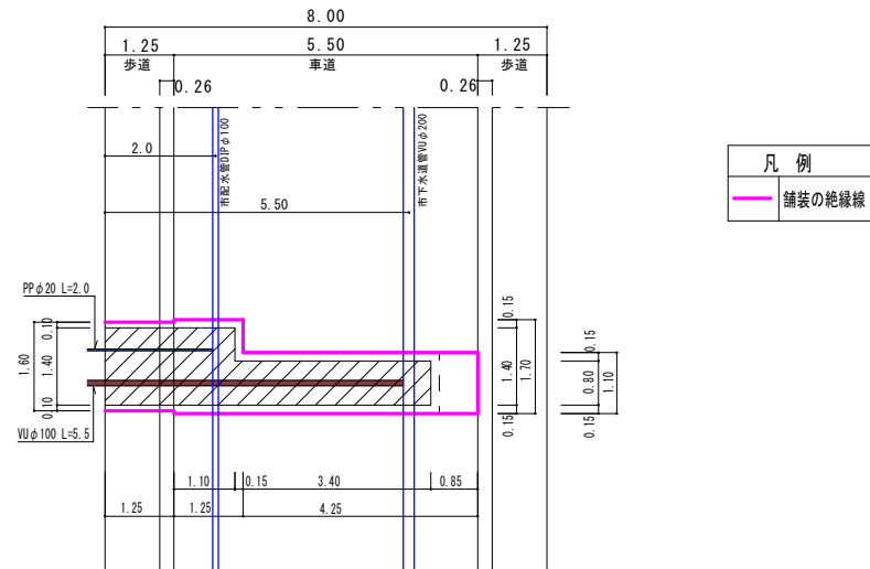
平面図 1:100
