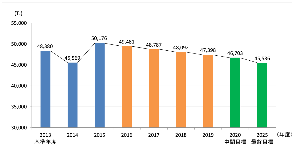
図4. 産業部門における目標とする推移
