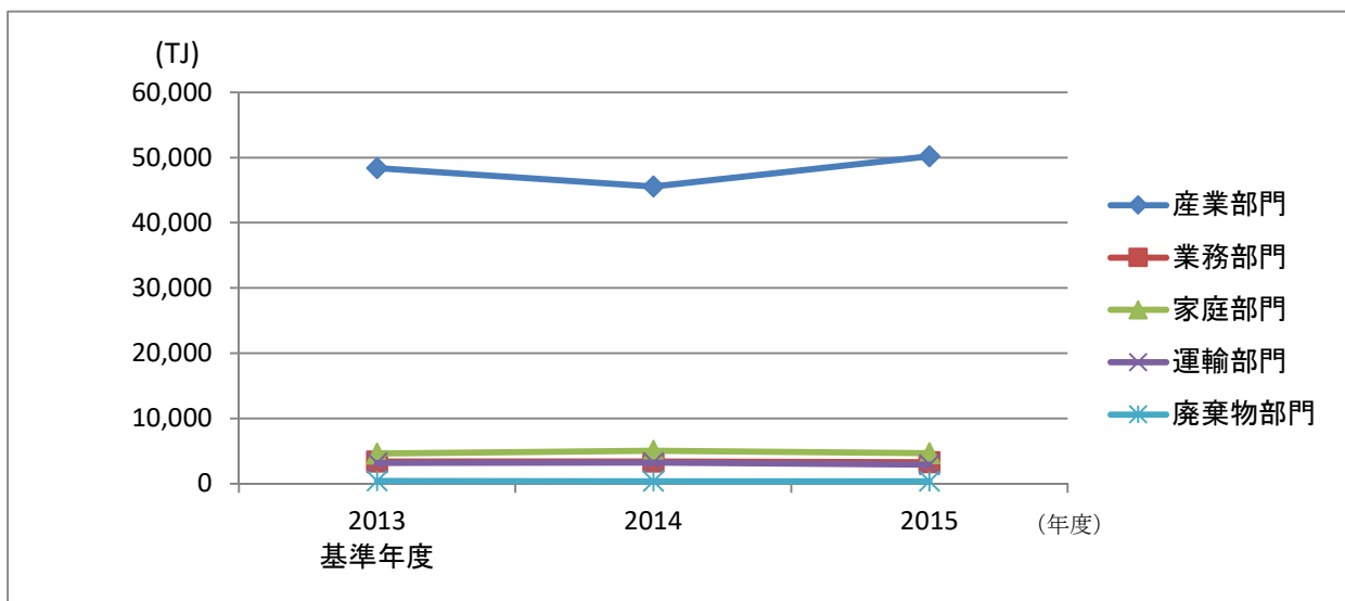
図3. エネルギー消費量の推移 (部門別)
