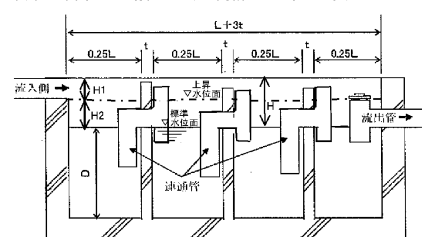
図-2 4槽式独立槽形阻集器の隔壁の設置位置
