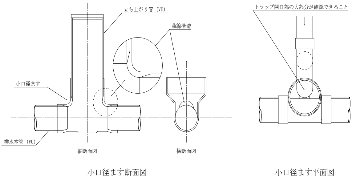
図 2-4-2 塩ビ枳
