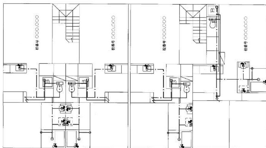
2階平面図
