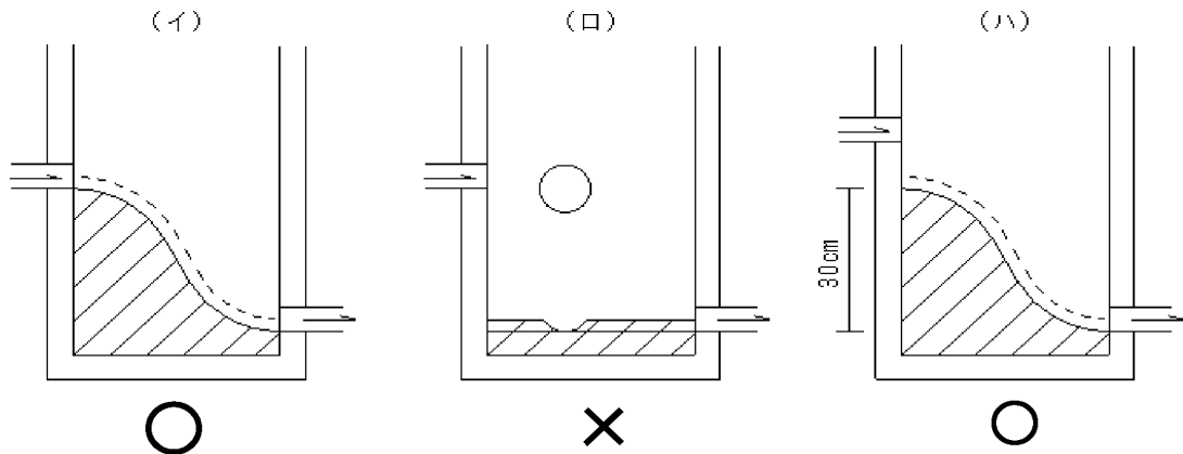
図 3-2-1 インバート
