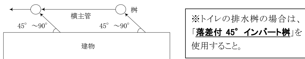
図 2-3-2 屋外横主管と枝管
