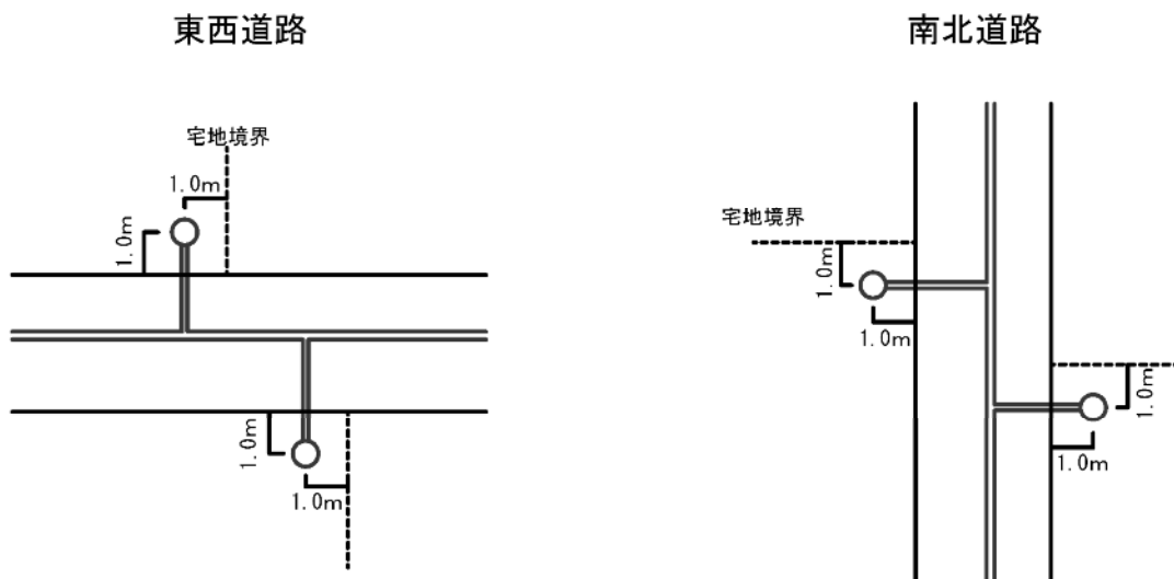
図 2-2-1 公共枿の設置位置(基本)
