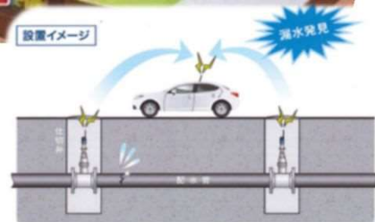
漏水音監視イメージ
