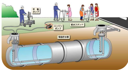
緊急貯水槽の概要図
