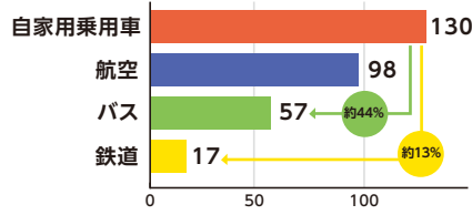
輸送量当たりの二酸化炭素の排出量(旅客) CO 2 排出原単位[g-CO 2 /人km](2019年度)
